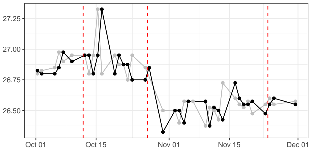
FSC-A
