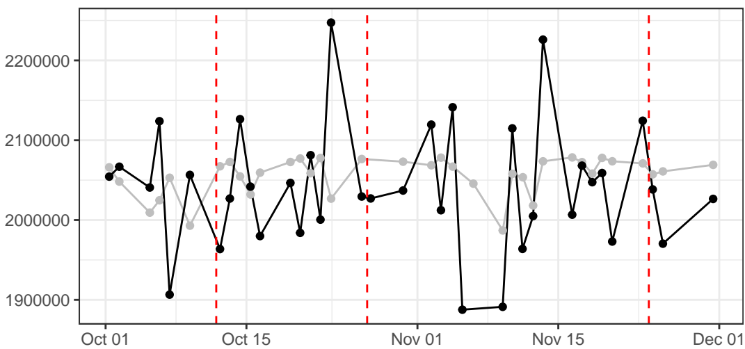
FSC-A
