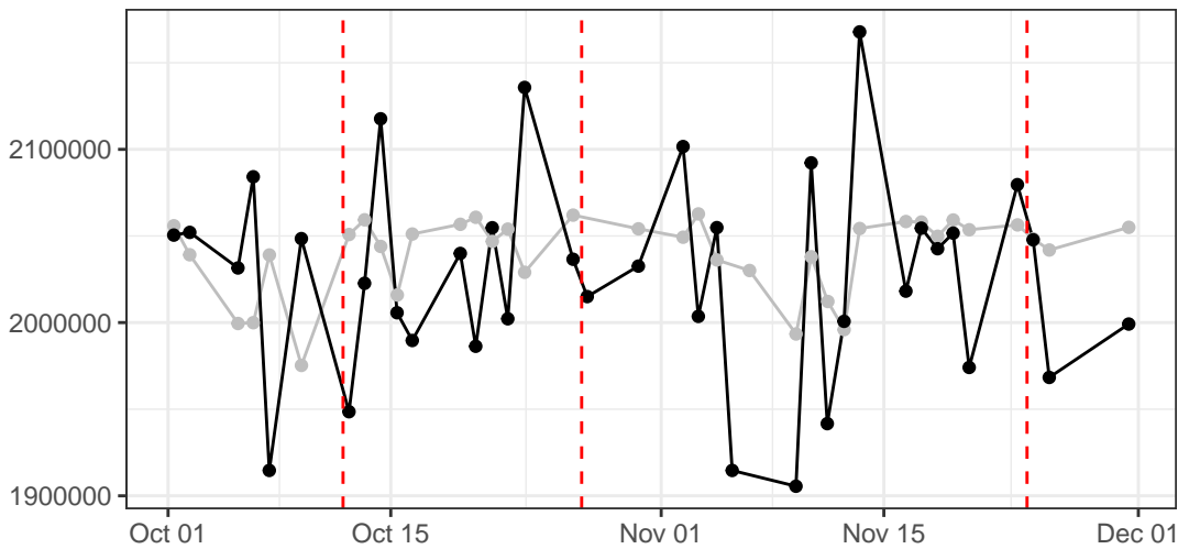
SSC-A
