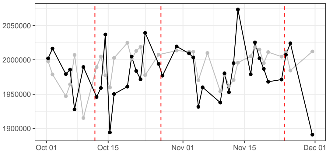
SSC-B-A
