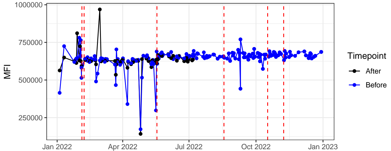
B7-A
