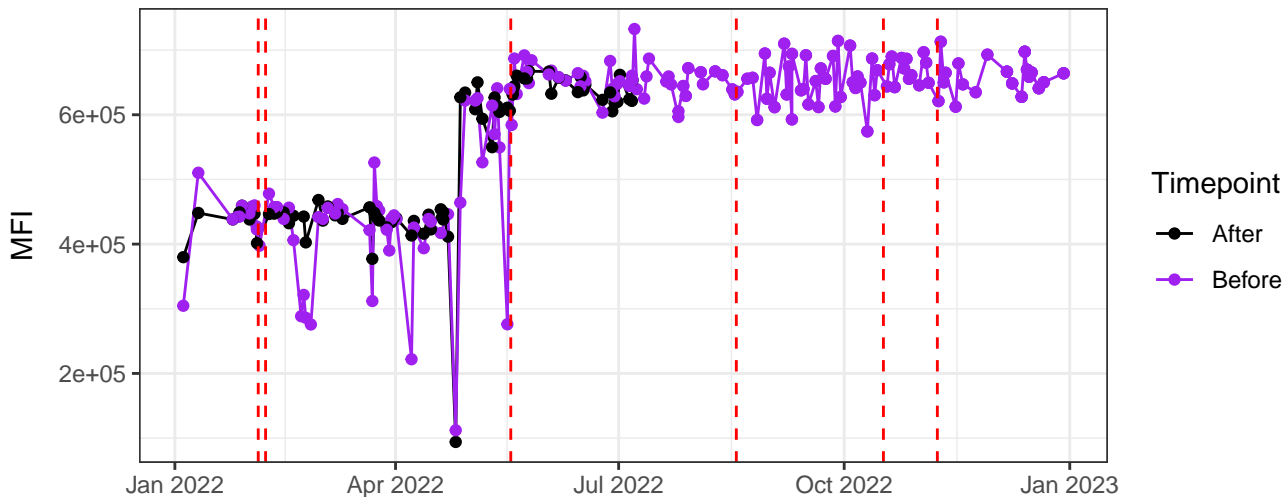
UV11-A
