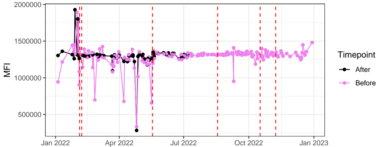
V5-A
