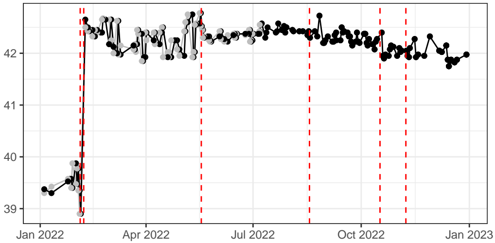
FSC-A
