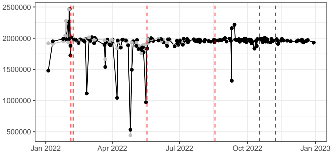
SSC-B-A
