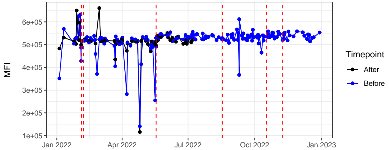
B6-A
