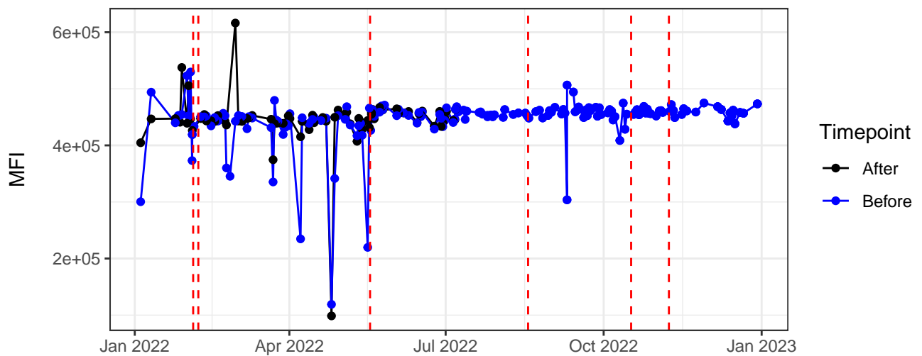
B7-A
