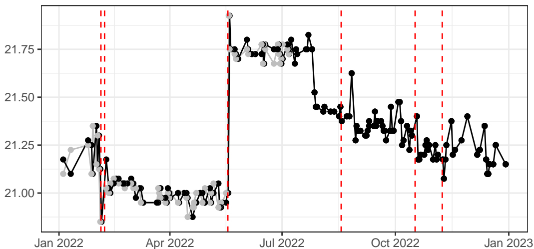
Red_LaserDelay
