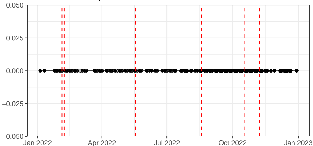
Red_LaserDelay
