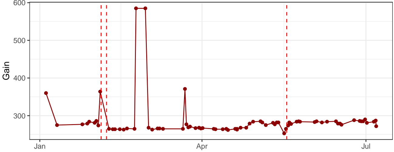
R4-A_Gain
