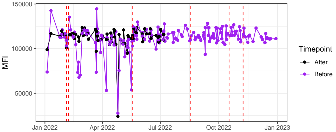
UV14-A
