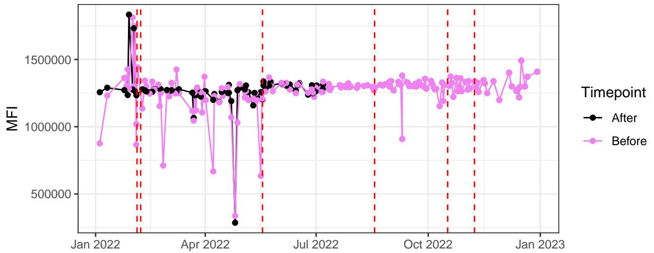
V4-A
