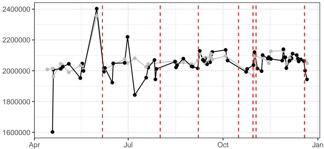
SSC-B-A
