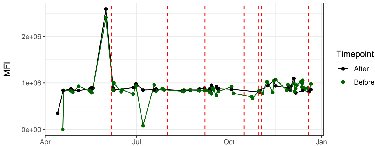
YG9-A
