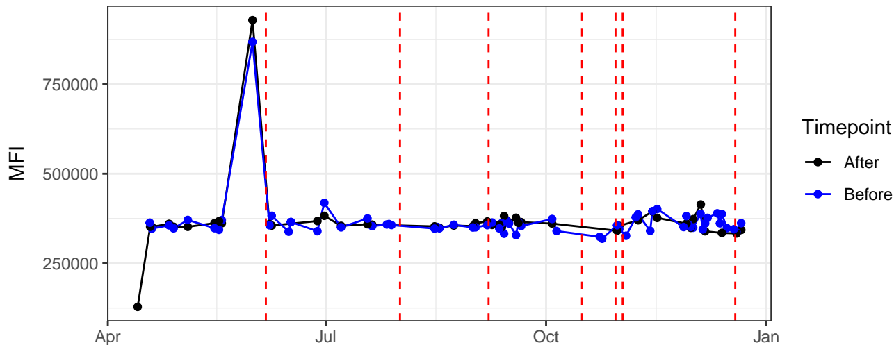
B12-A
