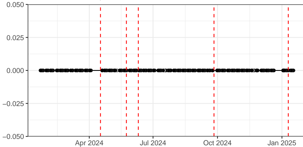
Red_LaserDelay
