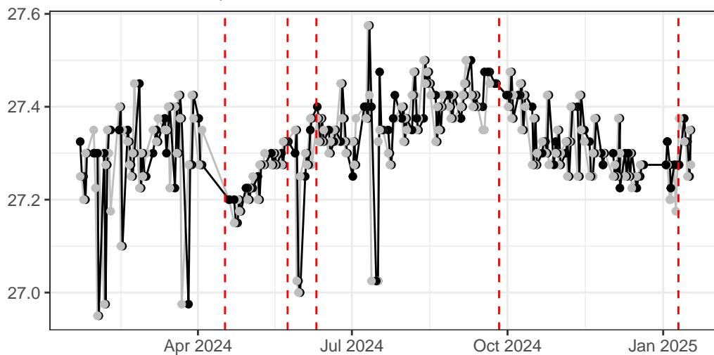
FSC-A
