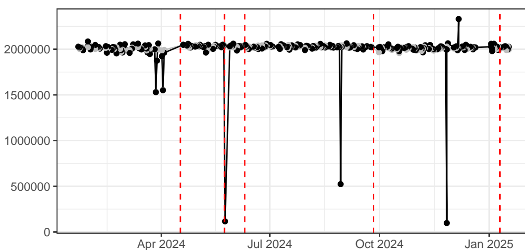
FSC-A
