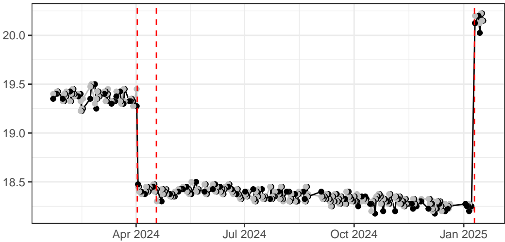
Red_LaserDelay
